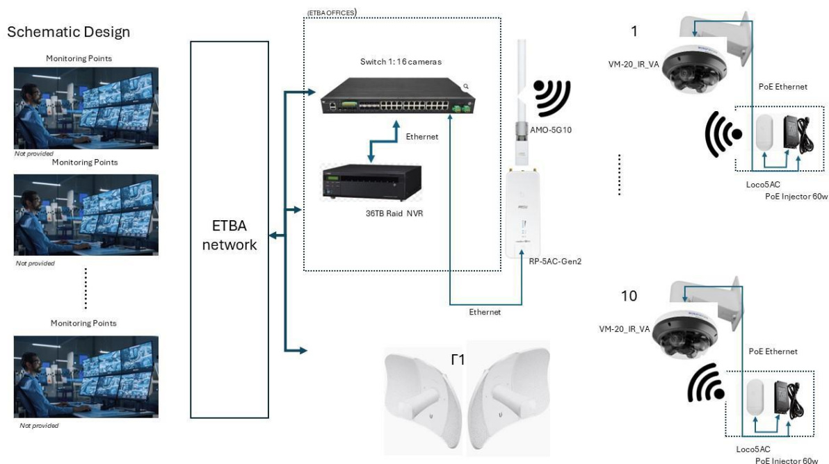
Εικόνα 3: Διάγραμμα σε σημεία με παροχή ρεύματος – Ε.Π. Κομοτηνής
